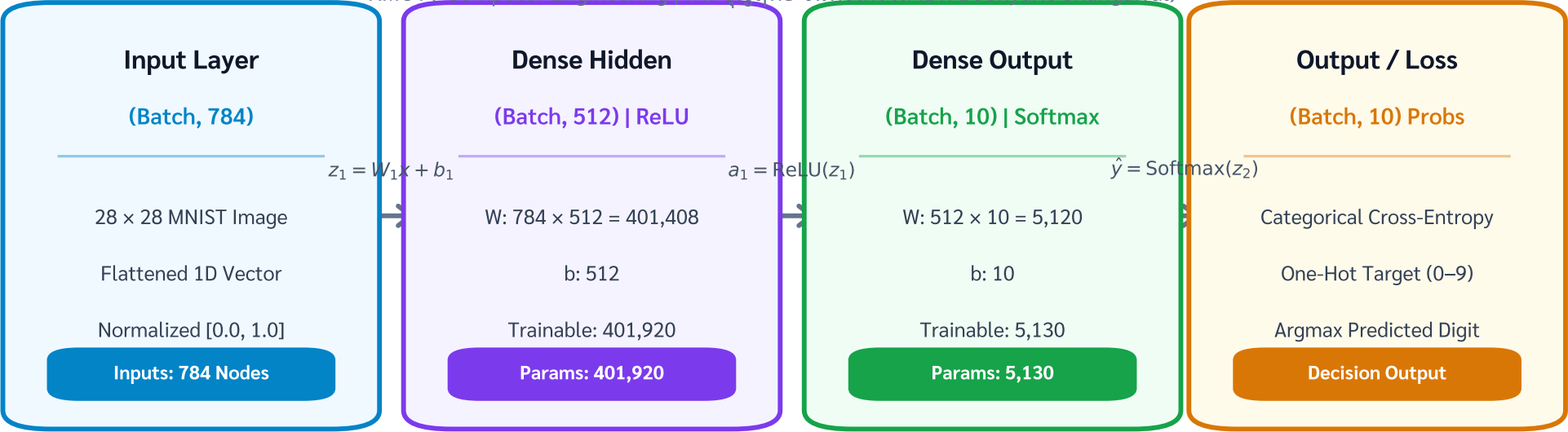
Figure 2: สถาปัตยกรรมโครงข่ายประสาทเทียมแบบเชื่อมต่อเต็มรูปแบบ (Baseline 2-Layer Fully-Connected DNN)
